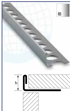
183S Προφίλ INOX ανοξειδωτος χάλυβας
