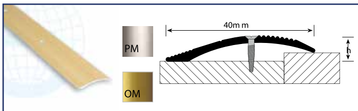
218A Προφίλ εξομάλυνσης δαπέδου από αλουμίνιο
