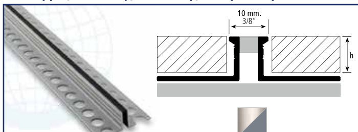
223A Αρμός διαστολής - συστολής αλουμινίου με καουτσούκ
