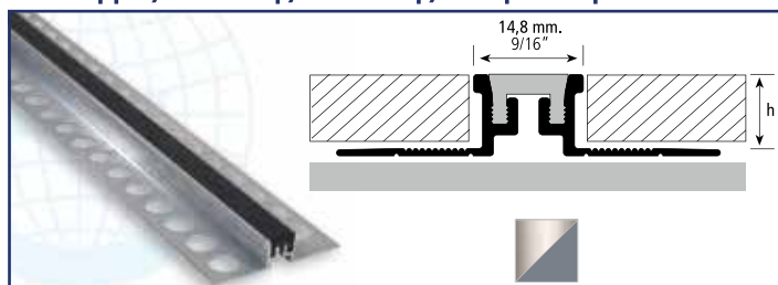
214A Αρμός διαστολής - συστολής αλουμινίου με καουτσούκ
