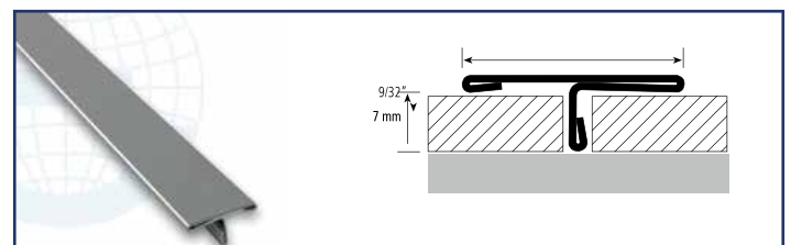
232S-IB Συνδετικός αρμός Ταψ ανοξείδωτος
